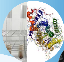
生合成
